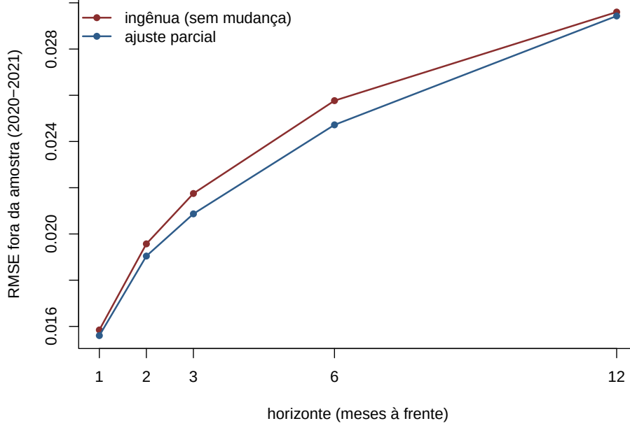
Figura 8: RMSE fora da amostra, ajuste parcial vs. ingênua, por horizonte de previsão.
